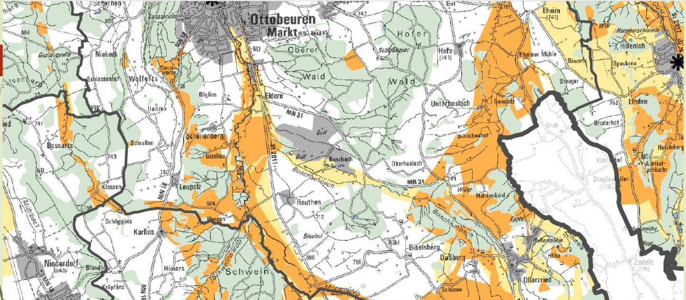
Einstufung des Konfliktpotenzials für die Nutzung mit großflächigen Freiflächen-Photovoltaikanlagen
